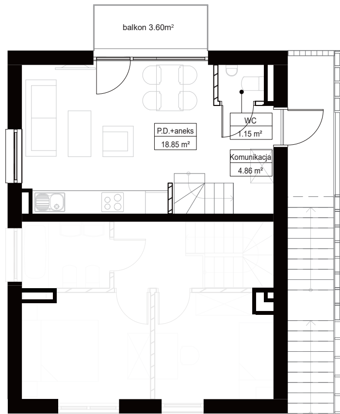
Poziom 1 wejście
